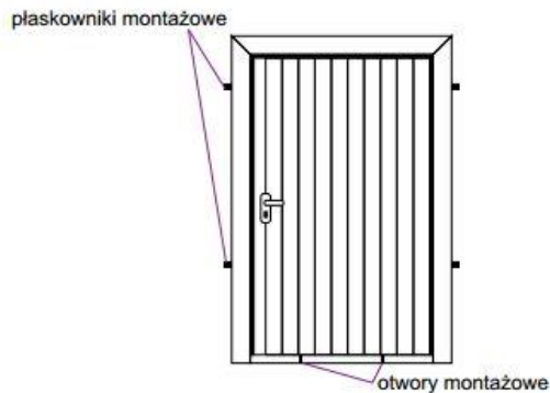
Rys. 1 montaż płaskowników montażowych
